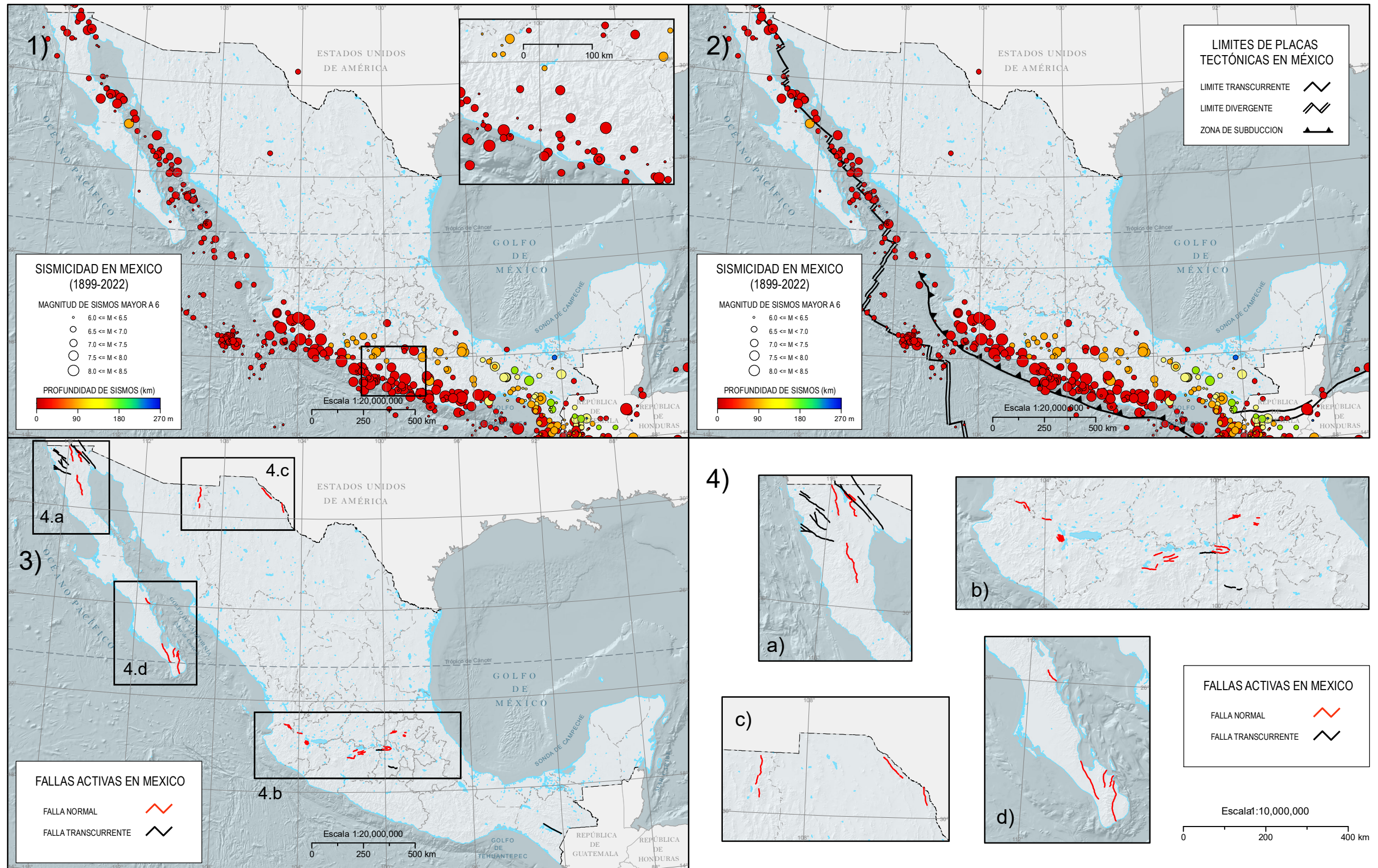
III.1.3.1 Sismos mayores a M6 en México (1899-2022) III.1.3.3 Fallas activas continentales en México
